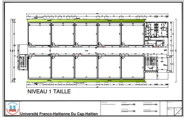
Figure 11 : Plan des 10 premières salles de classe qui seront construites sur le campus de Limonade.
